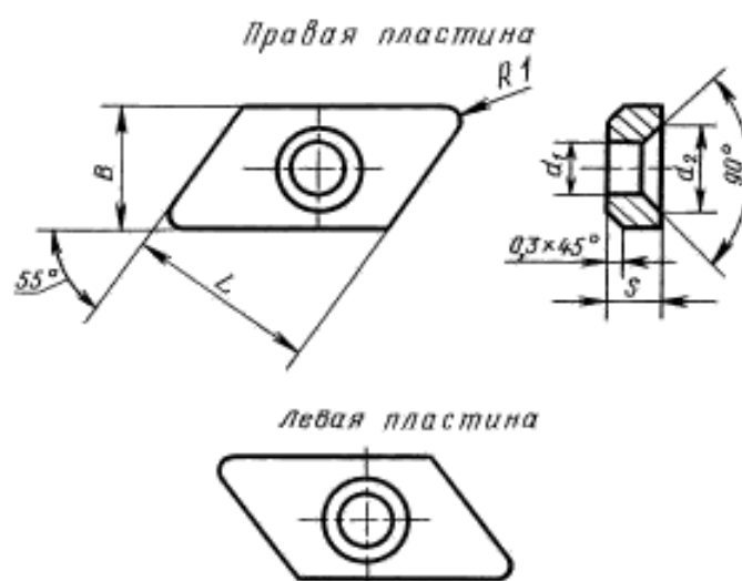
Размеры, мм
