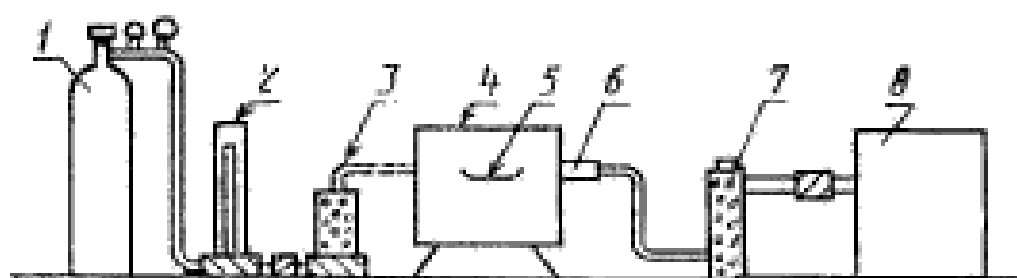
Рисунок 1 — Установка для определения углерода
