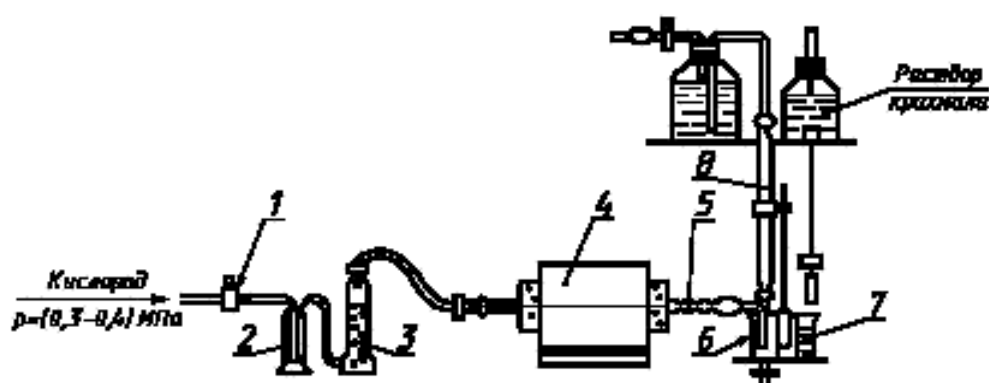
1 — кислородный баллон по ГОСТ 5583 с редукционным вентилем; 2 — склянка Тищенко, содержащая раствор марганцового кислого калия массовой концентрации 0,04 г/см 3 и раствор гидроксида калия массовой концентрации 0,4 г/см 3 ; 3 — сушильная колонка, заполненная хлористым кальцием; 4 — трубчатая печь с карборундовыми нагревателями; 5 — фарфоровая (высокоглиноземистая) трубка длиной 750—800 мм и внутренним диаметром 20—26 мм; 6 — сосуд для титрования; 7 — сосуд для сравнения; 8 — бюретка
