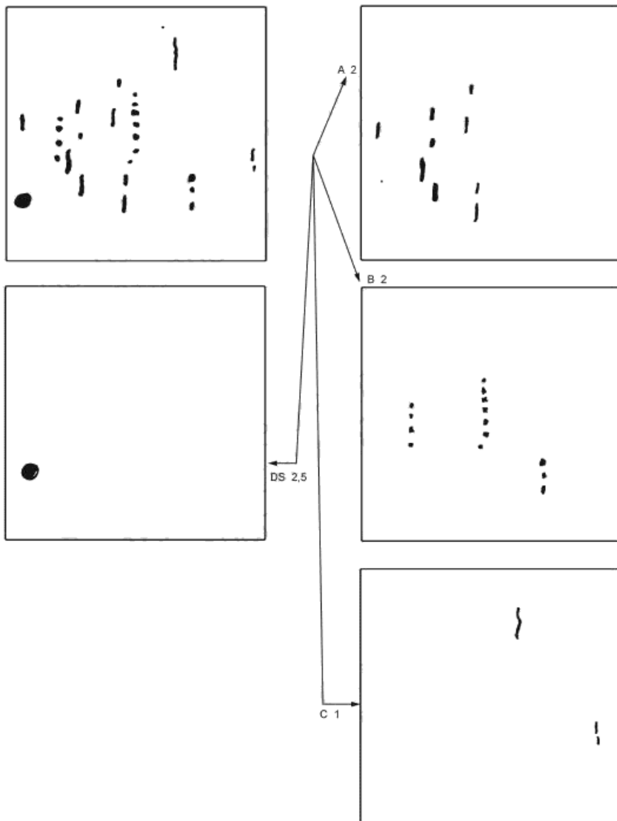
Рисунок В.1— Оценка поля
