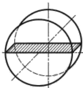
Рисунок 3 — Образец от прутка диаметром не более 25 мм
