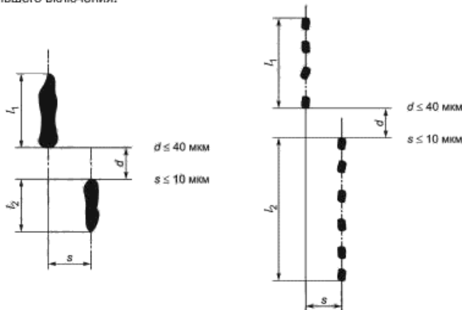
Рисунок 8 — Включения типов А и С
