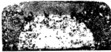
Трещины при осаживании заготовок в торец
