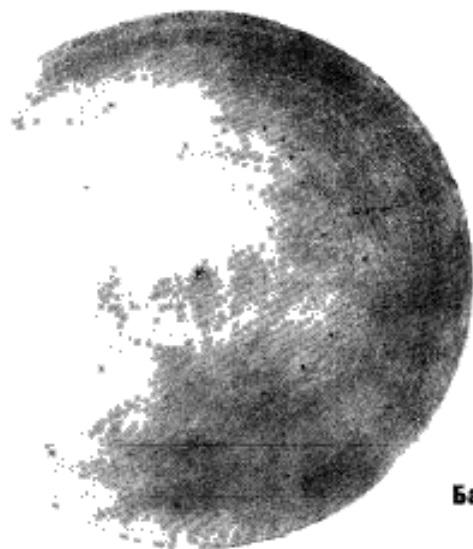
ШКАЛА № 1 Точечно-нитчатая неоднородность в макроструктуре сплавов после рафинирующих переплавов. Прутки размером 60—220 мм и переходные пробы.
