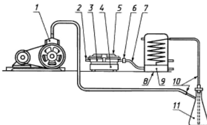
Установка для возгонки ртути
