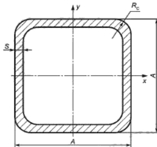
Рисунок А.1 — Форма профиля квадратных труб
